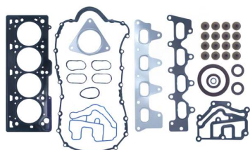
Full Gasket Set OEM No: 7701471886F Avortex No: 420
