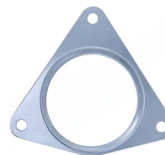
Exhaust Pipe Gasket OEM No: 7700423572 Avortex No: 426
