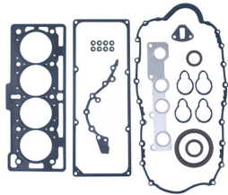
Full Gasket Set OEM No: 6001548043F Avortex No: 510
