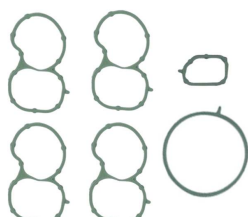
Intake Manifold Gasket OEM No: 71754211 Avortex No: 395
