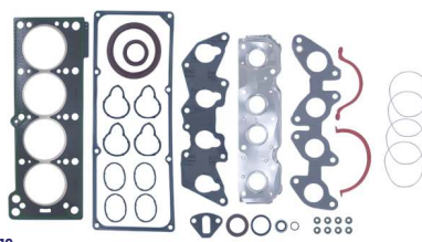
Full Gasket Set OEM No: 7701468709F Avortex No: 469
