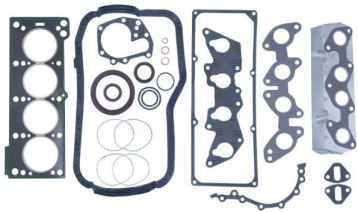
Full Gasket Set OEM No: 7701468142F Avortex No: 460
