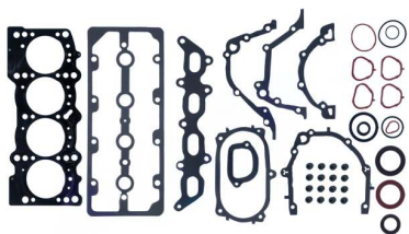
Full Gasket Set OEM No: 71716871 Avortex No: 280
