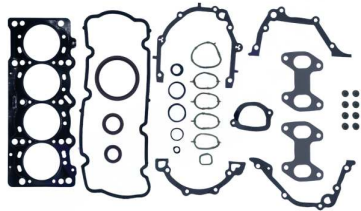
Full Gasket Set OEM No: 71718503F Avortex No: 262
