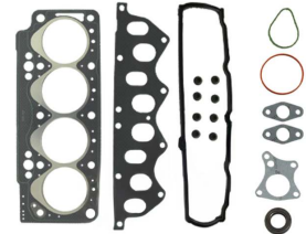
Cylinder Head Gasket Set OEM No: 7701468189 Avortex No: 491
