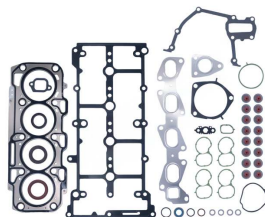
Full Gasket Set OEM No: 71769851F Avortex No: 380
