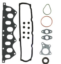
Zylinderkopfdichtungssatz ohne Zylinderkopfdich... OEM-Nr.: 7701468189 Avortex-Nr.: 4910S
