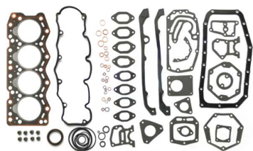
Vollständiger Dichtungssatz OEM-Nr.: 7701206361F Avortex-Nr.: 470
