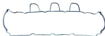
Ventildeckeldichtung OEM-Nr.: 7701070607 Avortex-Nr.: 438
