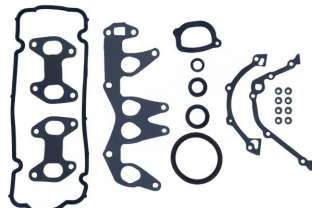
Vollständiger Dichtungssatz ohne Zylinderkopfdic... OEM-Nr.: 5893663 Avortex-Nr.: 2700S
