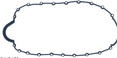
Ungekerbt Ölwannendichtung OEM-Nr.: 7700273486 Avortex-Nr.: 445
