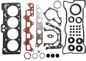
Vollständiger Dichtungssatz OEM-Nr.: 04111-16120 Avortex-Nr.: 6050701
