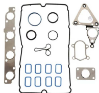
Zylinderkopfdichtungssatz ohne ZKD OEM-Nr.: XS4Q 6008 AA Avortex-Nr.: 6049702
