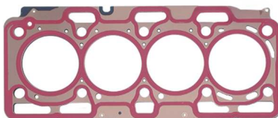
Zylinderkopfdichtung OEM-Nr.: 110447055R Avortex-Nr.: 703
