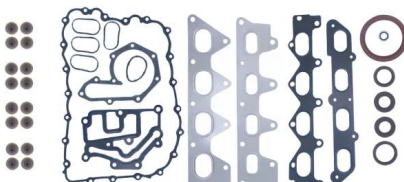
Vollständiger Dichtungssatz ohne Zylinderkopfdic... OEM-Nr.: 7701471278F Avortex-Nr.: 5800S
