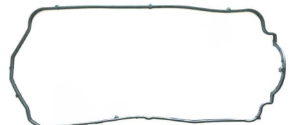
Ventildeckeldichtung OEM-Nr.: 7701059314 Avortex-Nr.: 455
