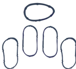
Ansaugkrümmerdichtung OEM-Nr.: 8200052311 Avortex-Nr.: 436
