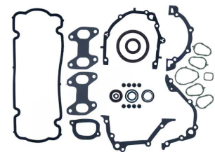
Vollständiger Dichtungssatz ohne Zylinderkopfdic... OEM-Nr.: 71740296F Avortex-Nr.: 2690S
