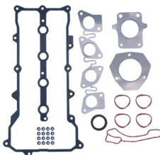
Zylinderkopfdichtungssatz ohne Zylinderkopfdich... OEM-Nr.: 101012709R Avortex-Nr.: 7210S
