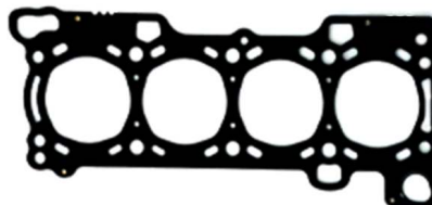
1,30mm 3 Loch Zylinderkopfdichtung OEM-Nr.: 500387069 Avortex-Nr.: 607
