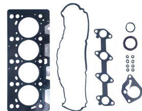
Zylinderkopfdichtungssatz OEM-Nr.: 7701473371 Avortex-Nr.: 402
