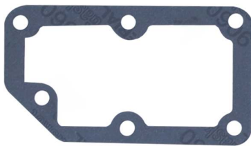
R-12 Wasserpumpendichtung (klein - Kesik) OEM-Nr.: N/A Avortex-Nr.: 1821512
