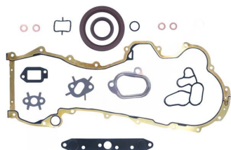
Kurbelgehäusedichtungssatz OEM-Nr.: 71744286 Avortex-Nr.: 230
