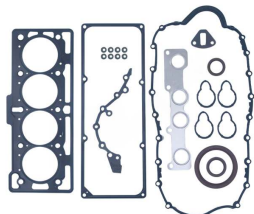
Vollständiger Dichtungssatz OEM-Nr.: 6001548043F Avortex-Nr.: 510
