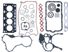
Vollständiger Dichtungssatz OEM-Nr.: 7701475278F Avortex-Nr.: 480
