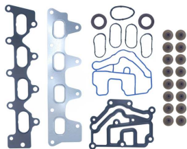
Zylinderkopfdichtungssatz ohne Zylinderkopfdich... OEM-Nr.: 7701471886 Avortex-Nr.: 4210S
