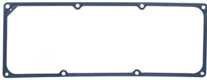
Ventildeckeldichtung OEM-Nr.: 7701471719 Avortex-Nr.: 464
