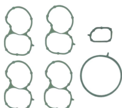
Ansaugkrümmerdichtung OEM-Nr.: 71754211 Avortex-Nr.: 395
