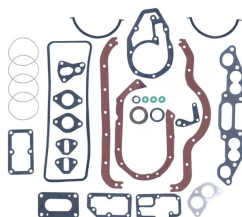
Motor-Dichtungssatz ohne Zylinderkopfdichtung OEM-Nr.: 7701458694 Avortex-Nr.: 5400S
