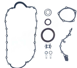
Kurbelgehäusedichtungssatz OEM-Nr.: 7701473371A Avortex-Nr.: 414
