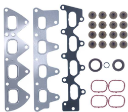
Zylinderkopfdichtungssatz ohne Zylinderkopfdich... OEM-Nr.: 7701474372 Avortex-Nr.: 5910S
