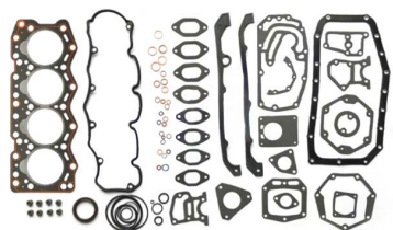
Vollständiger Dichtungssatz OEM-Nr.: 71728336F Avortex-Nr.: 610
