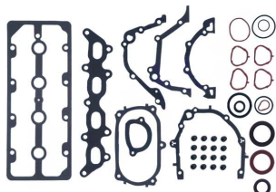
Vollständiger Dichtungssatz ohne Zylinderkopfdic... OEM-Nr.: 71716871 Avortex-Nr.: 2800S
