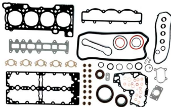
Vollständiger Dichtungssatz OEM-Nr.: 504049360F Avortex-Nr.: 602
