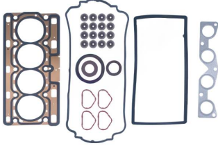
Full Takım Conta OEM No: 7701473003 Avortex No: 450
