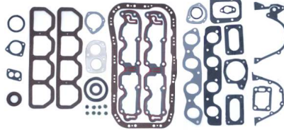
Full Takım Conta SKC Hariç OEM No: 5893330 Avortex No: 3600S
