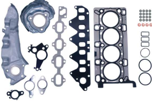
Üst Takım Conta OEM No: 101015474R Avortex No: 801
