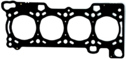
1,20mm 2 Delik Silindir Kapak Conta OEM No: 500387068 Avortex No: 606
