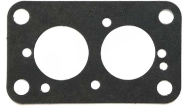
Karbüratör Ara Conta OEM No: N/A Avortex No: 1831314
