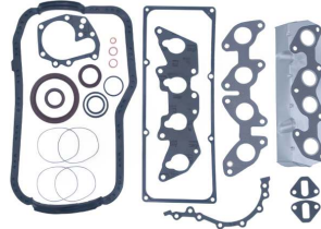
Full Takım Conta SKC Hariç OEM No: 7701468142F Avortex No: 4600S
