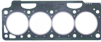
Silindir Kapak Conta OEM No: 7700859273 Avortex No: 572
