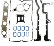
Motor Takım Conta SKC hariç OEM No: 2S7Q 6008 AA Avortex No: 6049101
