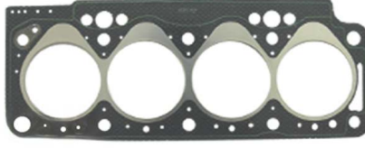
1.80 3 Delik Silindir Kapak Conta OEM No: 7700860266 Avortex No: 494
