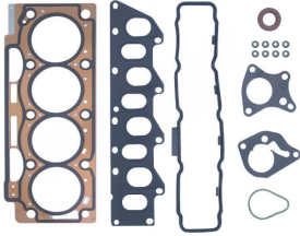
Full Takım Conta OEM No: 7701470288F Avortex No: 430
