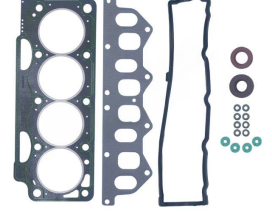
Üst Takım Conta OEM No: 7701467058 Avortex No: 571
