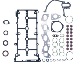
Full Takım Conta SKC Hariç OEM No: 71769851S Avortex No: 381
