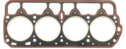
Silindir Kapak Conta OEM No: 4338254 Avortex No: 5131020
