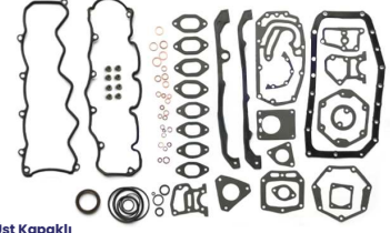
Full Takım Conta SKC Hariç OEM No: 71728336 Avortex No: 6100SU
