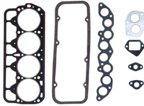
Üst Takım Conta OEM No: 5880442U Avortex No: 345
