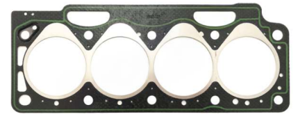
1.60 2 Delik Silindir Kapak Conta OEM No: 7700107818 Avortex No: 501
