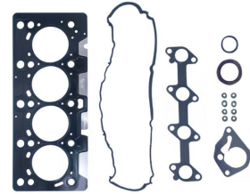
Üst Takım Conta OEM No: 7701473371 Avortex No: 402
