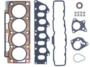
Üst Takım Conta OEM No: 7701470288 Avortex No: 431
