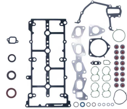
Full Takım Conta SKC Hariç OEM No: 71769851CF Avortex No: 383
