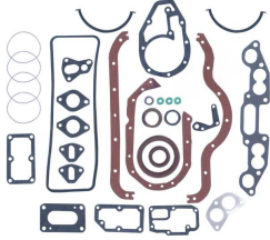
Full Takım Conta SKC Hariç OEM No: 7701460627 Avortex No: 5410S
