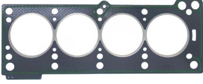
Silindir Kapak Conta OEM No: 7700739302 Avortex No: 462
