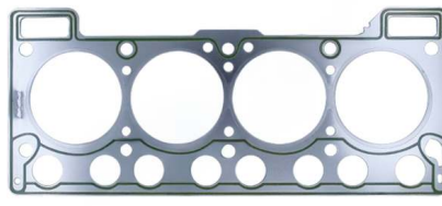
Saç Takıyeli Silindir Kapak Conta OEM No: 7700680689 Avortex No: 532
