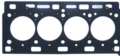
Silindir Kapak Conta OEM No: 8200459643 Avortex No: 482
