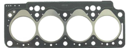
1.401 Delik Silindir Kapak Conta OEM No: 7700860265 Avortex No: 492
