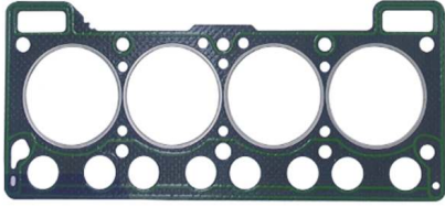
Silikonlu Silindir Kapak Conta OEM No: 7700680689 Avortex No: 531
