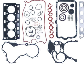
Full Takım Conta OEM No: 7701475278F Avortex No: 480
