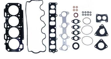
Üst Takım Conta OEM No: 71718658 Avortex No: 221
