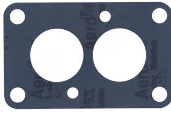
Karbüratör Ara Conta OEM No: N/A Avortex No: 1821414
