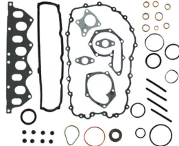
Full Takım Conta SKC Hariç OEM No: 7701468189F Avortex No: 4900S
