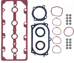
Üst Takım Conta SKC Hariç OEM No: 71749165 Avortex No: 6510S
