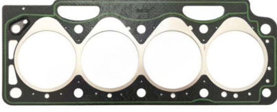
1.40 1 Delik Silindir Kapak Conta OEM No: 7701039398 Avortex No: 500
