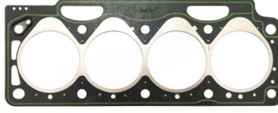
1.80 3 Delik Silindir Kapak Conta OEM No: 7701039399 Avortex No: 502
