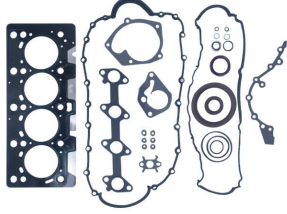
Viton Keçeli Subap Lastikli Full Takım Conta OEM No: 7701473371F Avortex No: 401
