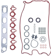
Üst Takım Conta SKC Hariç OEM No: 7701475278 Avortex No: 4810S
