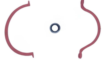
Karter Boğaz Lastik Conta OEM No: 7700867315 Avortex No: 467
