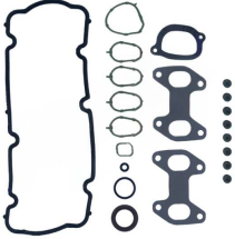
Üst Takım Conta SKC Hariç OEM No: 71718503 Avortex No: 2600S
