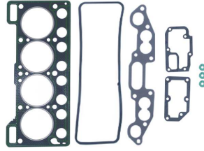
Üst Takım Conta OEM No: 7701458694U Avortex No: 543
