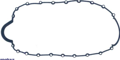
Tırnaksız Karter Conta OEM No: 7700273486 Avortex No: 445
