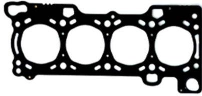
1,30mm 3 Delik Silindir Kapak Conta OEM No: 500387069 Avortex No: 607
