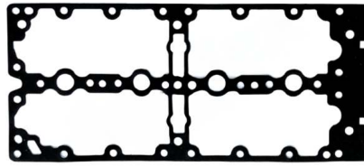
Üst Kapak Conta OEM No: 504052452 Avortex No: 637
